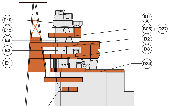
IJN Aoba 1945
